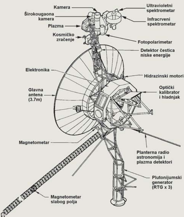
INŽENJERSKO REMEK- -DELO: Konstrukcija Vojadžera
