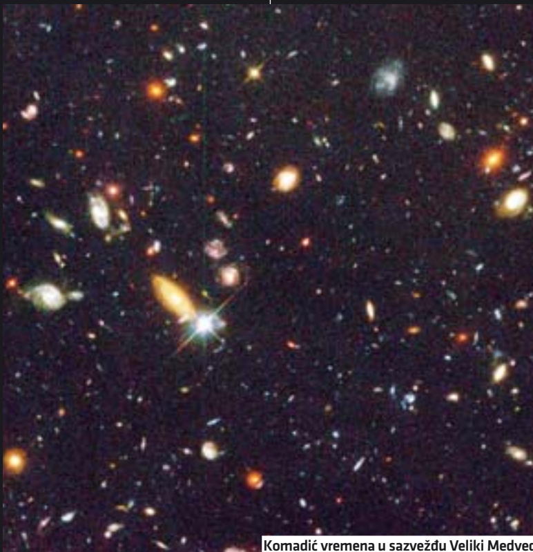
Komadić vremena u sazvežđu Veliki Medved
